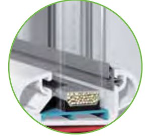
20-24-32 mm Cam Uygulamaları 20-24-32 mm Glass Application Применение двойного и тройного стеклопакета
